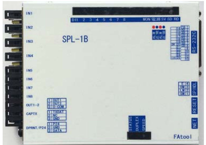
外形寸法 150X110X25 (mm)
